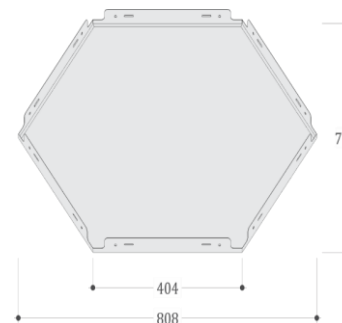
TẤM TRẦN LỤC GIÁC PHẪNG
