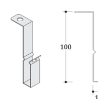
MÓC C38
