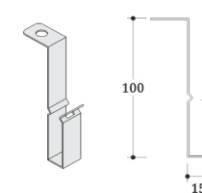
MÓC C38
