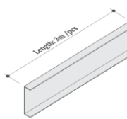
KHUNG C38
