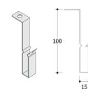
MÓC C38
