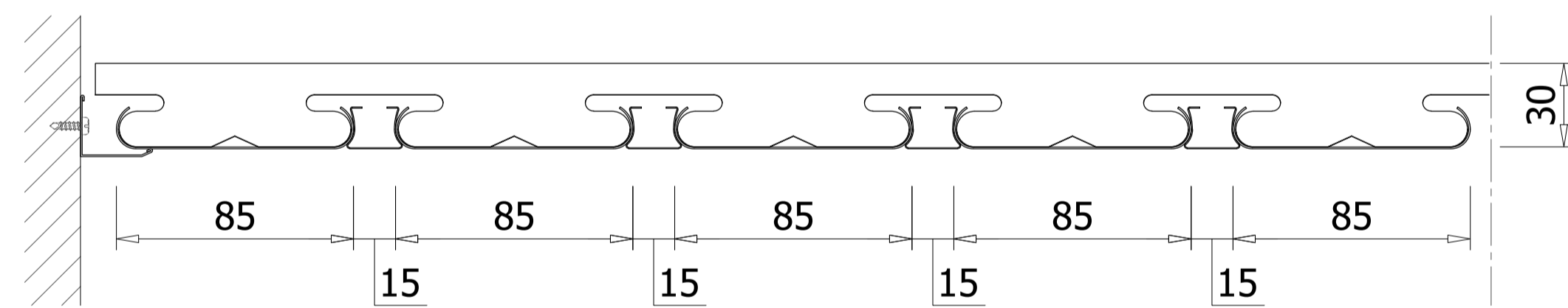
TYPICAL SECTION/ MẶT CẮT ĐIỂN HÌNH:
