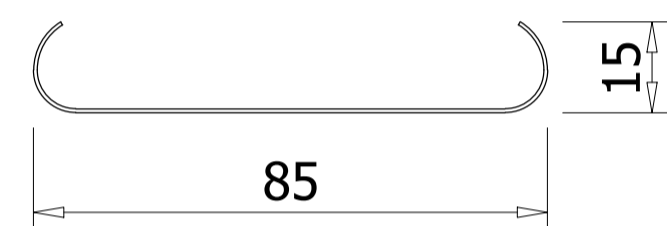
PANEL SECTION MẶT CẮT TẮM
