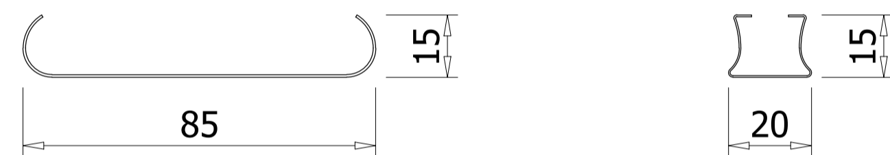
PANEL SECTION MẶT CẮT TẤM
